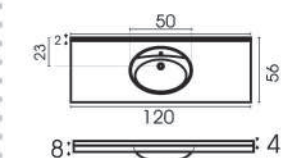
MIRAGE 120 120 x 56 x 8cm
