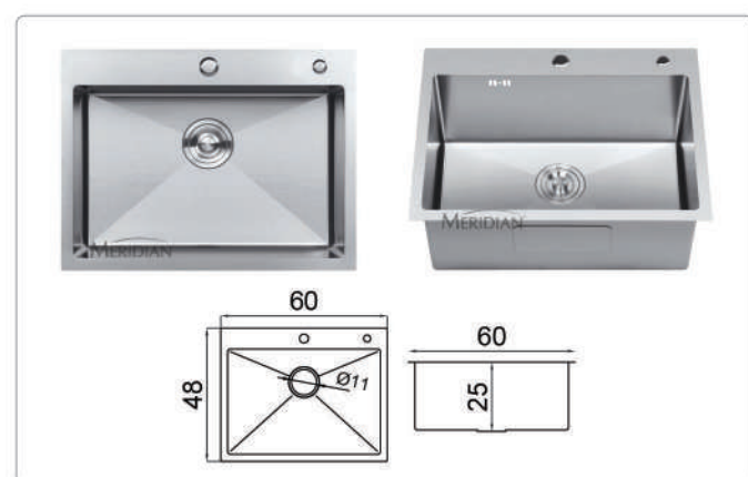
MX - 6048 (60 x 48 x 25cm) Silk
