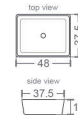
W - 8032 48 x 37.5 x 13cm
