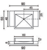
CORINA 90 x 55 x 20cm
