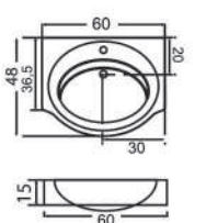
LINK 60 60 x 48 x 15cm
