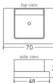
WM - 8065 70 x 48 x 24cm
