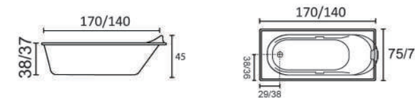
A ( 170 x 75 x 38cm ) B ( 140 x 70 x 37cm )
