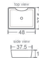
W - 8072A 48 x 37.5 x 13cm
