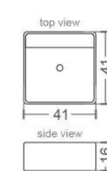
W - 8065 41 x 41 x 16cm
