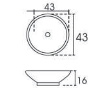
BONIA 43 x 16cm
