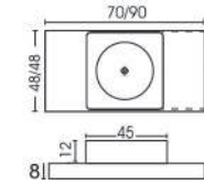
DURAFI 70 / 90 A : 70 x 48 x 20cm B : 90 x 48 x 20cm
